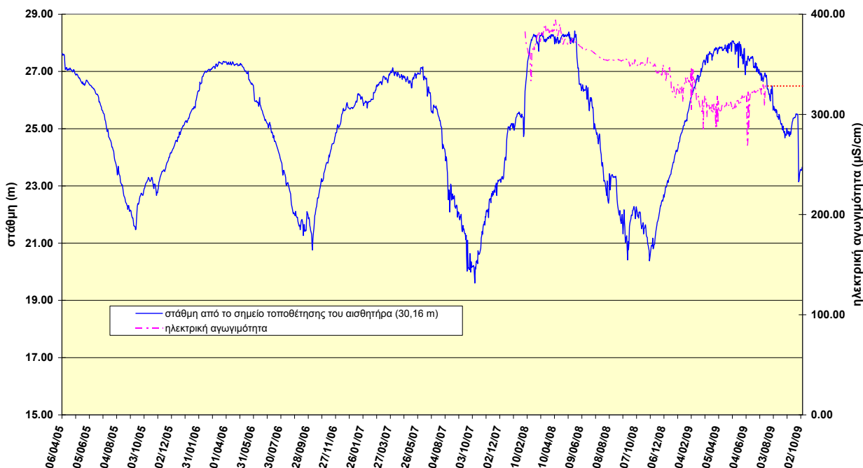
Εικόνα 10. Διάγραμμα διακύμανσης στάθμης και μεταβολής ηλ. αγωγιμότητας του σταθμού Κολενίου (..... περίοδος κατά την οποία το αισθητήριο ήταν εκτός λειτουργίας)
