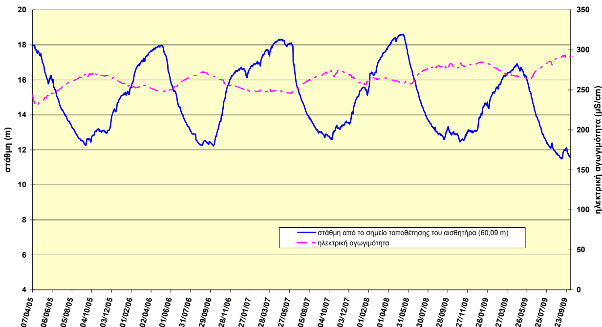
Εικόνα 11. Διάγραμμα διακύμανσης στάθμης και μεταβολής ηλεκτρικής αγωγιμότητας του σταθμού Αγιάς
