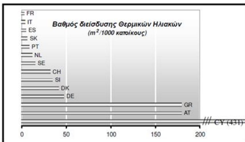
Σχήμα 4.7 Βαθμός διείσδυσης Ηλιακών Συλλεκτών Ελλάδα, 2002 [14]
