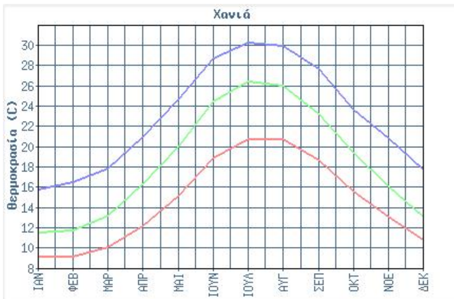
Διάγραμμα Μέγιστης, Ελάχιστης και Μέσης μηνιαίας θερμοκρασίας στα Χανιά
