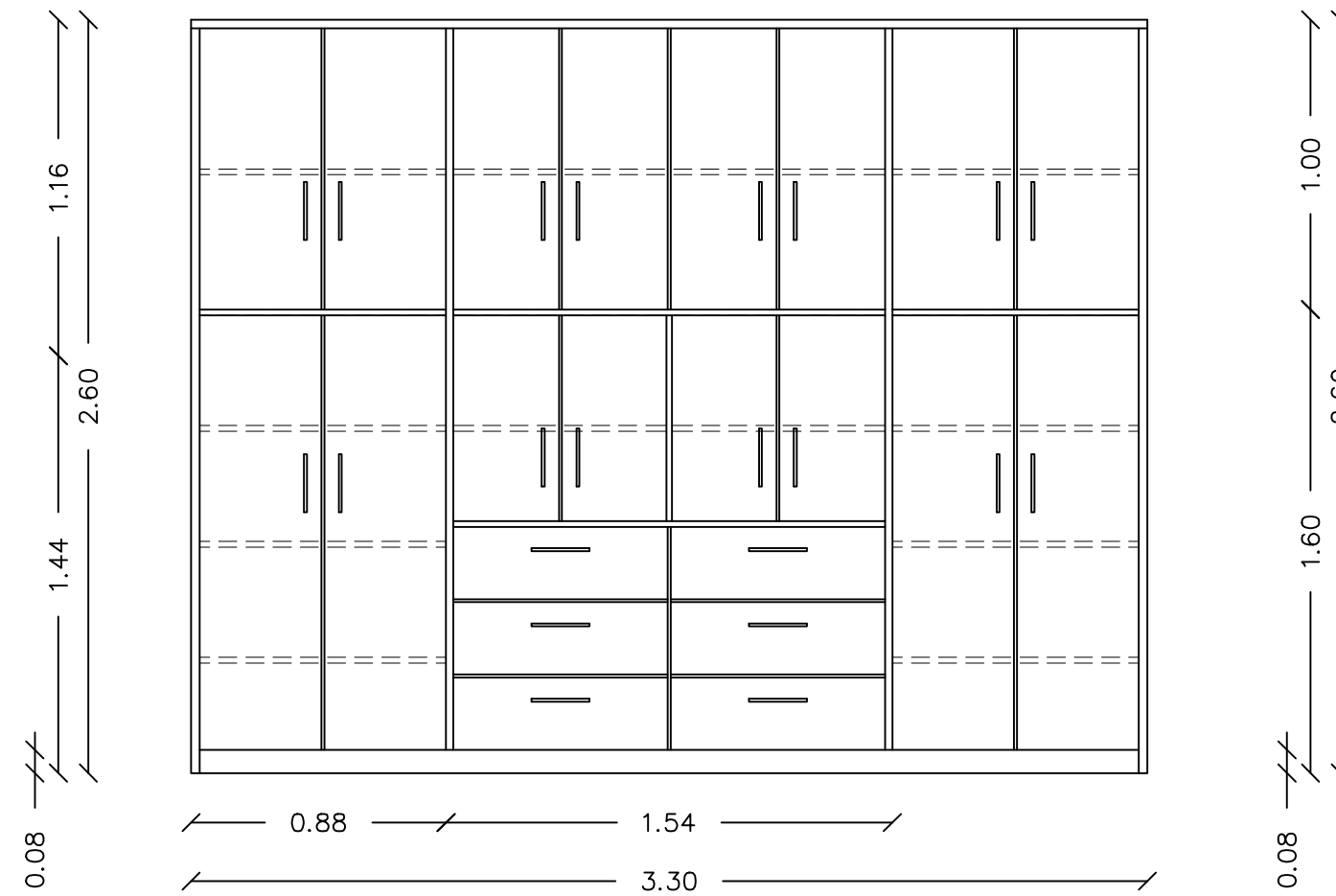
Ιματιοθήκη αίθουσας ύπνου κάτω κτιρίου
