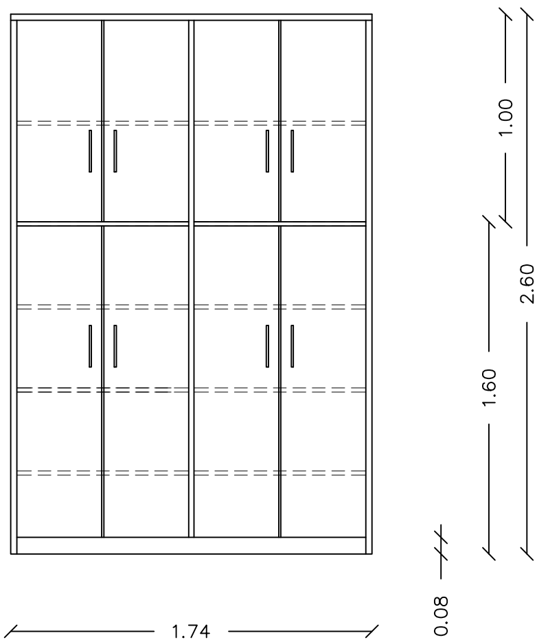
Ιματιοθήκη αίθουσας μόνωσης
