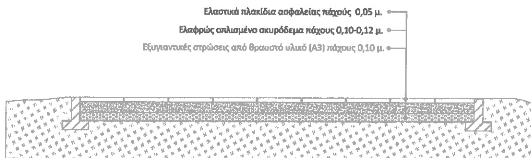
Εικόνα: Διατομή ενδεικτικής εφαρμογής δαπέδου ασφαλείας
