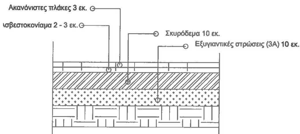
Τομή ενδεικτικής εφαρμογής ακανόνιστων πλακών από φυσικό υλικό
