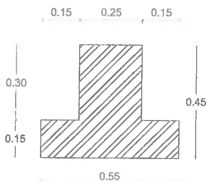
Εικόνα: Διατομή τοιχίου
