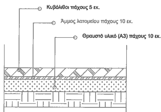
Εικόνα: Τομή ενδεικτικής εφαρμογής κυβόλιθου.
