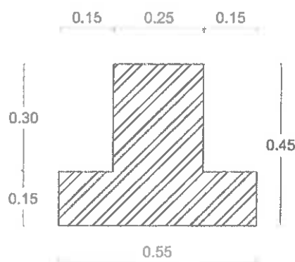
Εικόνα: Διατομή τοιχείου
