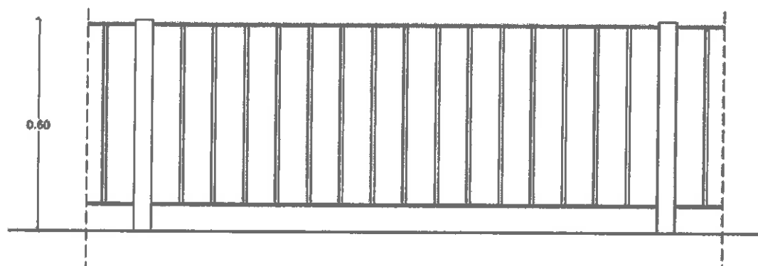
Εικόνα: Προτεινόμενη διάταξη μεταλλικής περίφραξης
